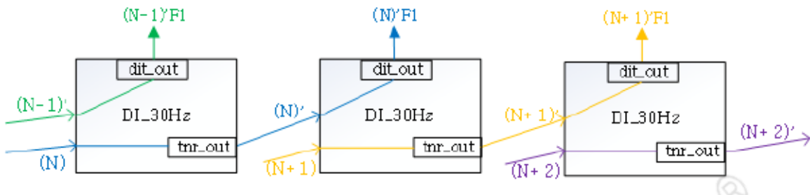
图 2-12: 30Hz 时序数据流
