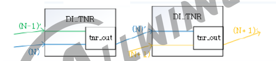
图 2-17: dit tnr 时序数据流
