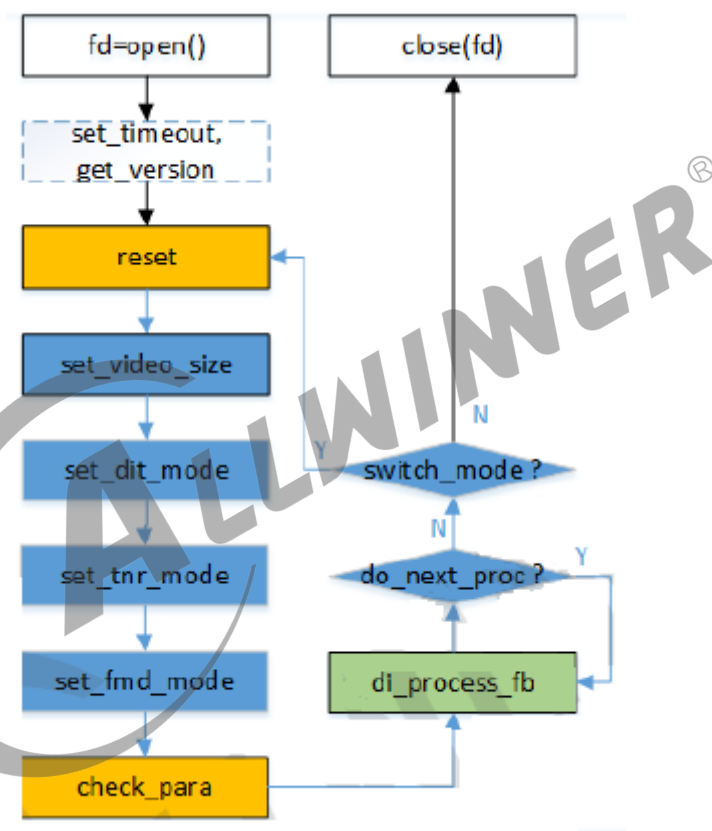
图 2-5: 驱动调用流程
