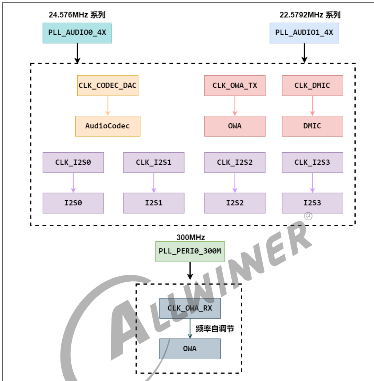
图 6-11: 时钟树 sun55iw6
