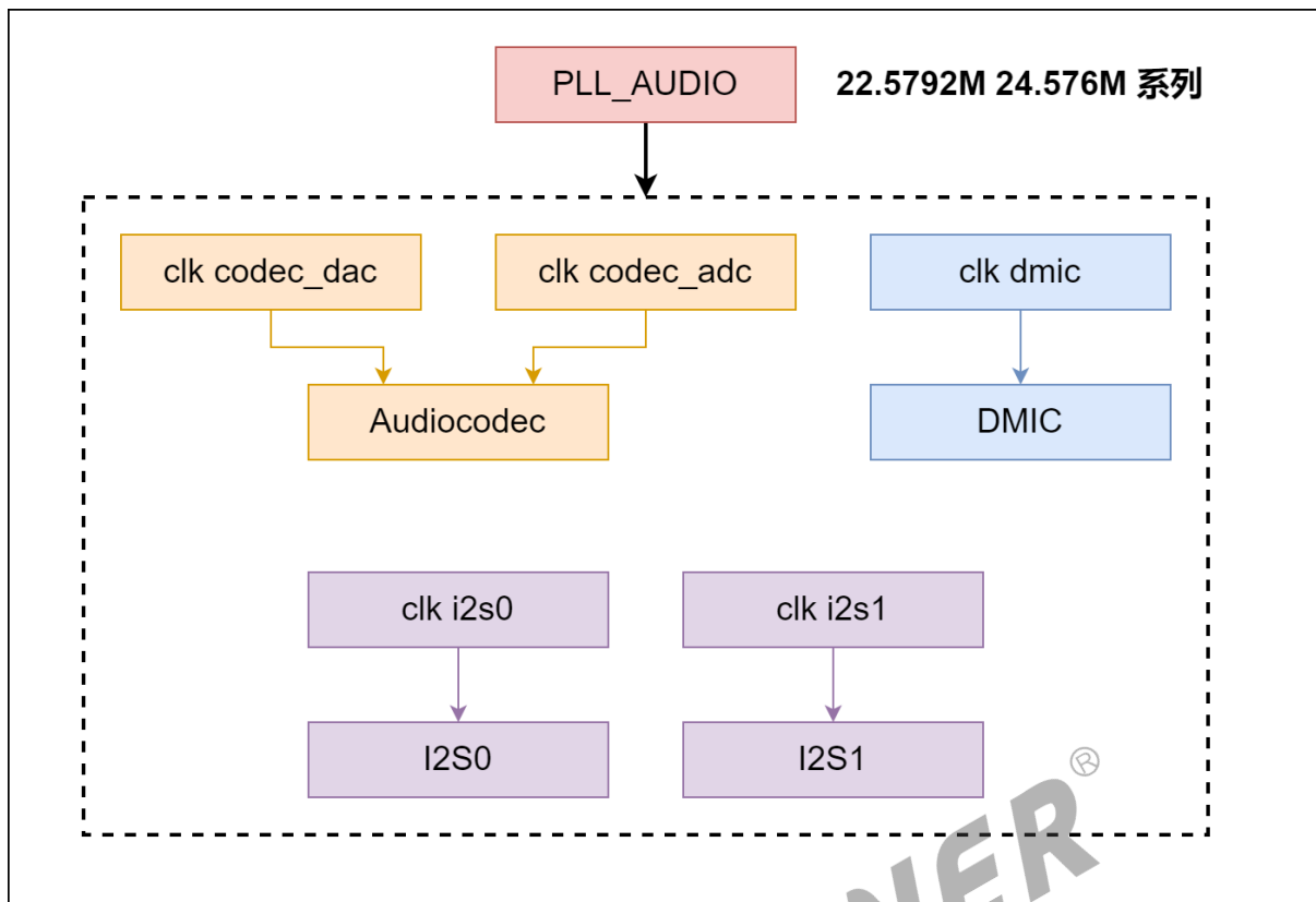
图 6-5: 时钟树 sun8iw21
