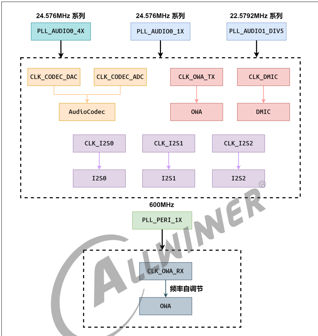
图 6-13: 时钟树 sun251iw1
