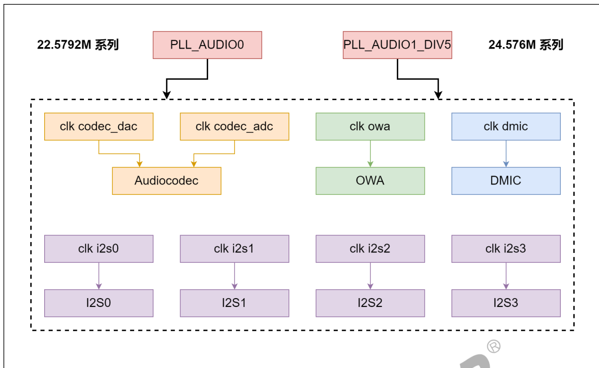
图 6-4: 时钟树 sun8iw20
