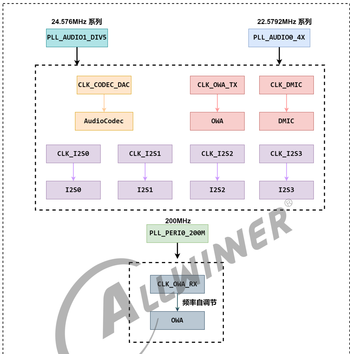
图 6-14: 时钟树 sun60iw2
