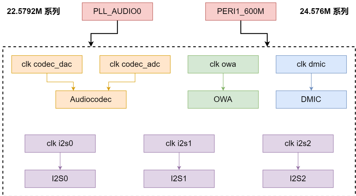
图 6-7: 时钟树 sun8iw22
