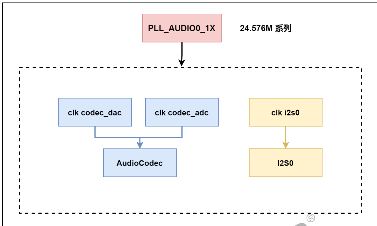
图 6-12: 时钟树 sun300iw1
