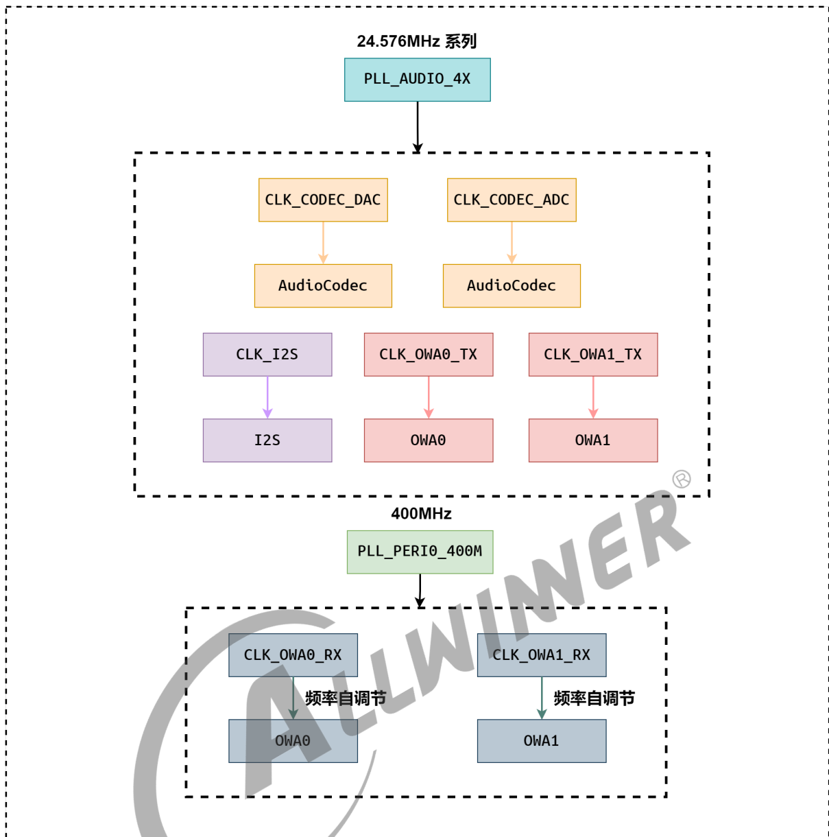
图 6-15: 时钟树 sun50iw15
