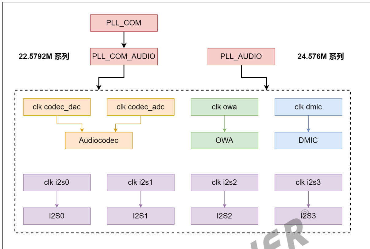
图 6-9: 时钟树 sun50iw10
