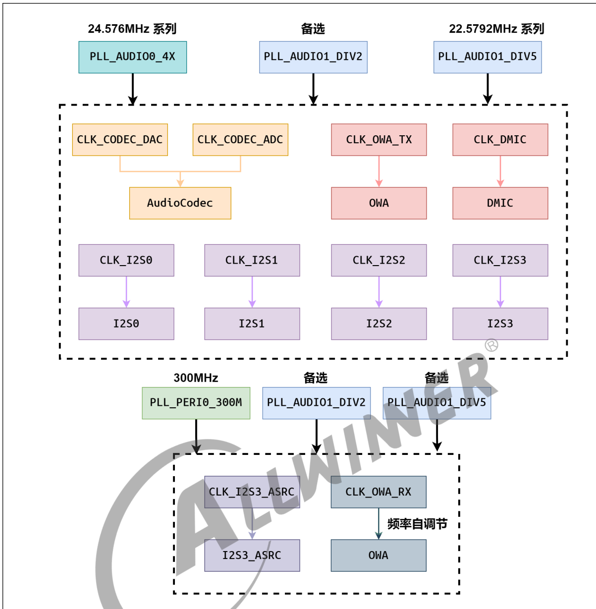
图 6-10: 时钟树 sun55iw3
