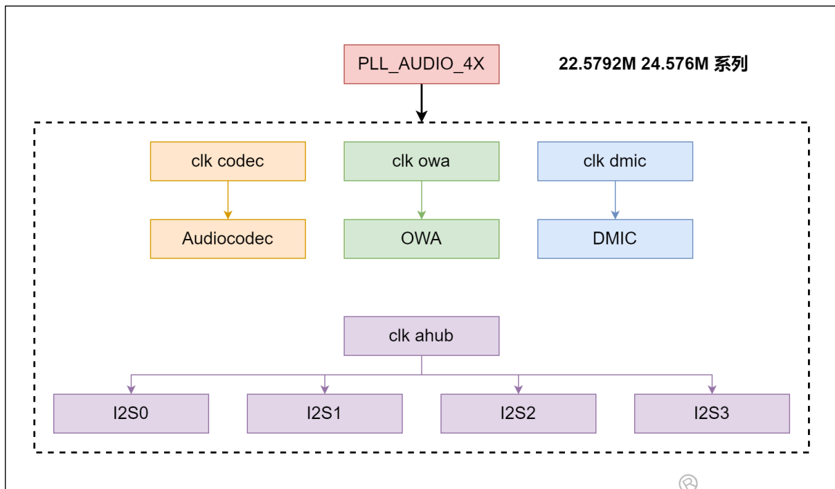
图 6-8: 时钟树 sun50iw9
