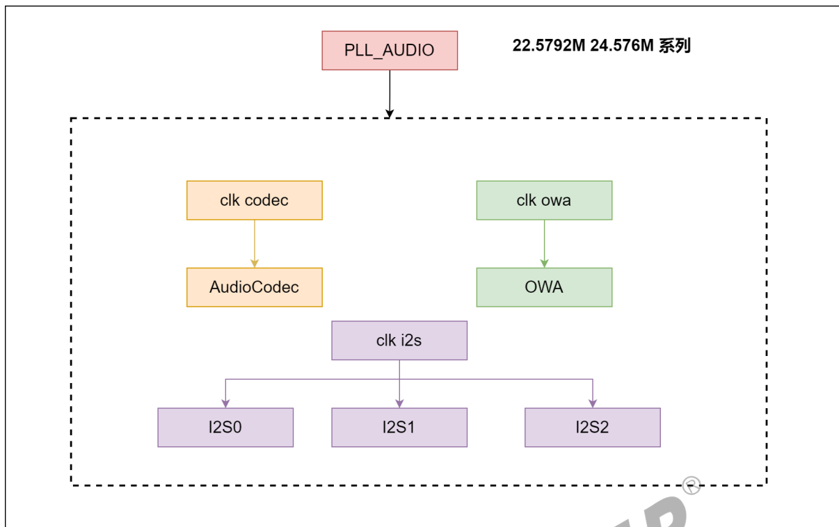
图 6-6: 时钟树 sun8iw11
