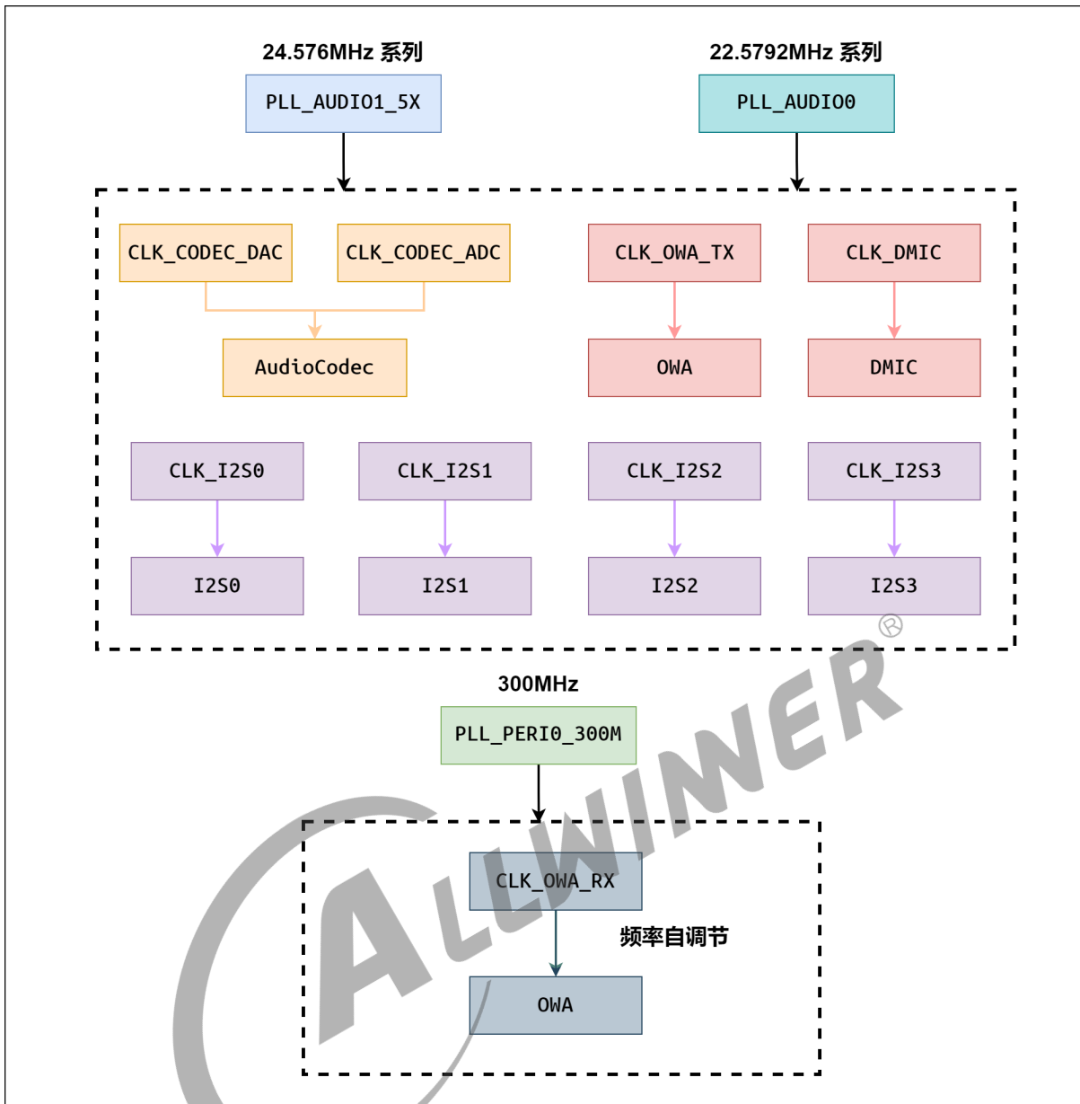
图 6-16: 时钟树 sun65iw1
