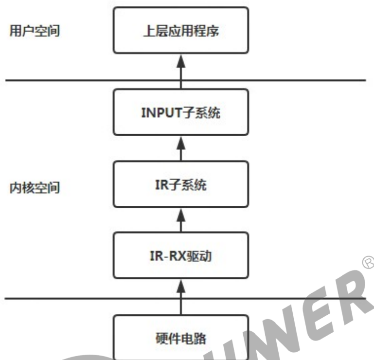
图 2-2: IR-RX 模块结构框图
