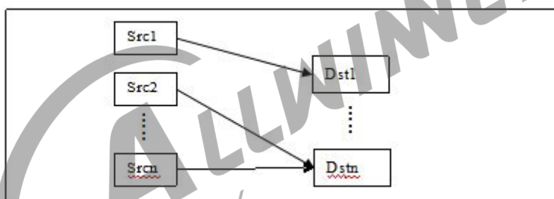
图 2-8: DMA Engine 散列拷贝示意图 (master 与 master)
